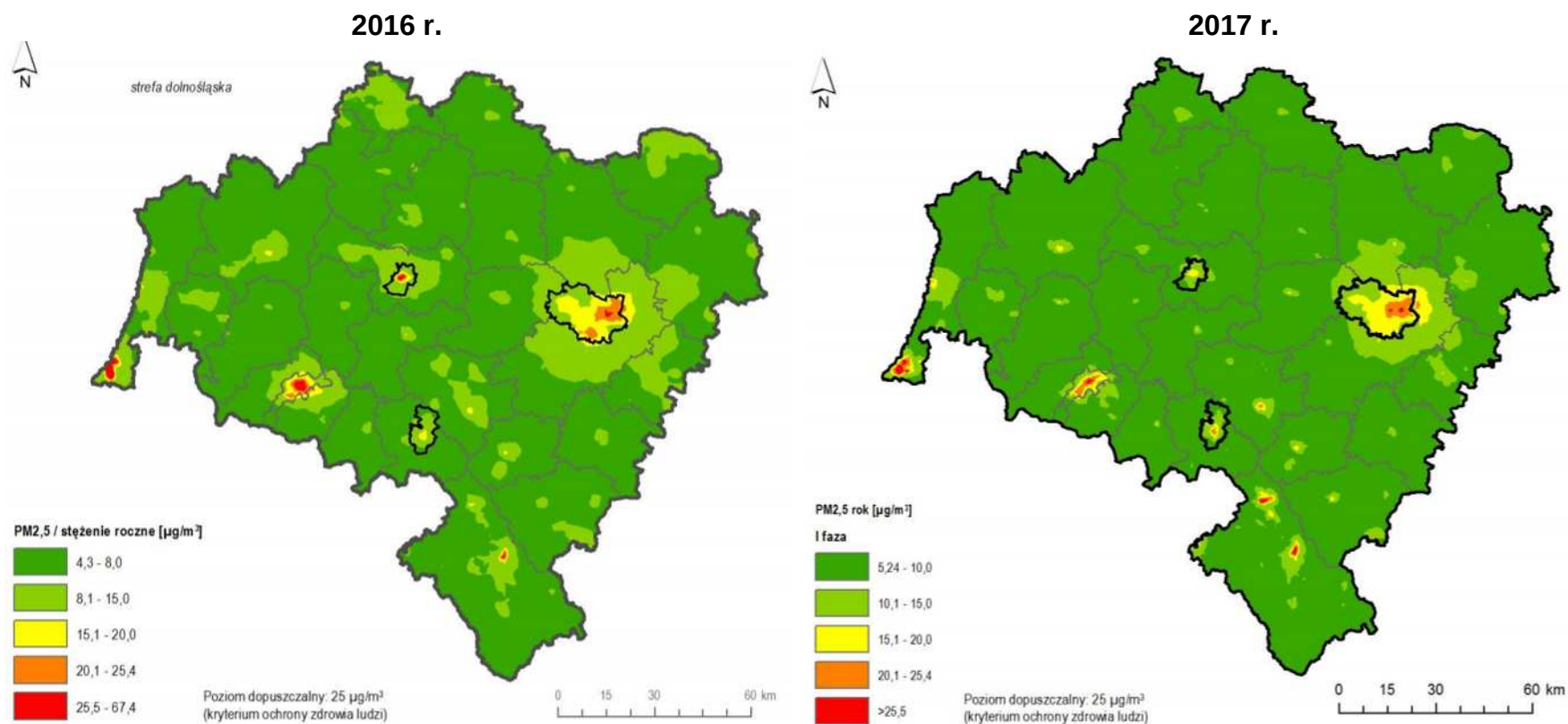
Rysunek 3.12 Rozkłady stężeń średniorocznych pyłu zawieszonego PM 2.5 na terenie województwa dolnośląskiego na podstawie wyników modelowania jakości powietrza opracowanych przez WIOŚ we Wrocławiu za 2016 i 2017 r. [59], [60]
