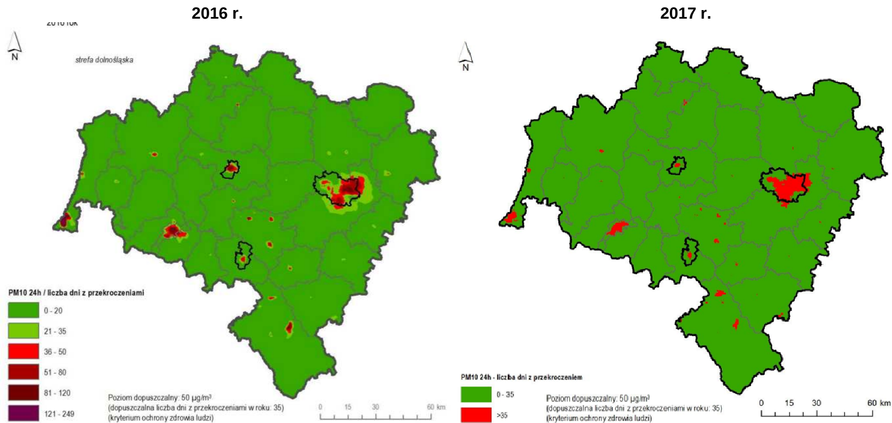
Rysunek 3.7 Rozkłady liczby dni z przekroczeniami dopuszczalnego poziomu 24-godzinnego pyłu zawieszonego PM 10 na terenie województwa dolnośląskiego na podstawie wyników modelowania jakości powietrza opracowanych przez WIOŚ we Wrocławiu za 2016 i 2017 r. [59], [60]
