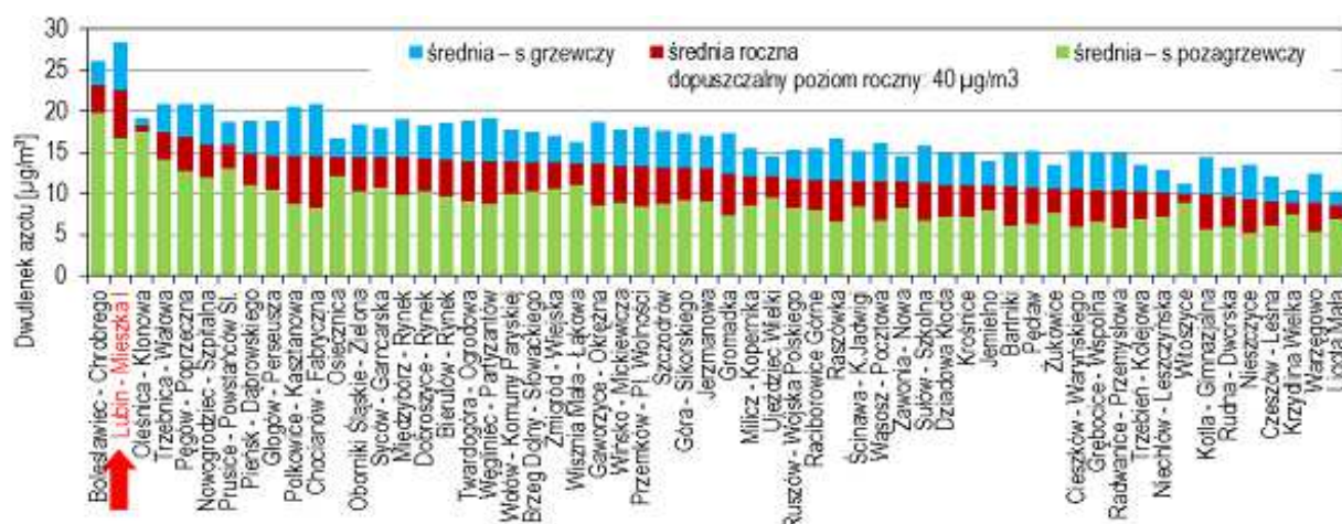
Rysunek 3.15 Poziomy stężen średniorocznych i sezonowych NO 2 na terenie woj. dolnośląskiego w 2013 r. – pomiary met. pasywną [WIOŚ]
