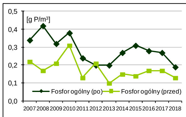
Rysunek 3.26 Niektóre parametry jakości wód rzeki Zimnicy przed i po zrzucie ścieków z oczyszczalni w latach 2007 – 2018 [MPWiK]
